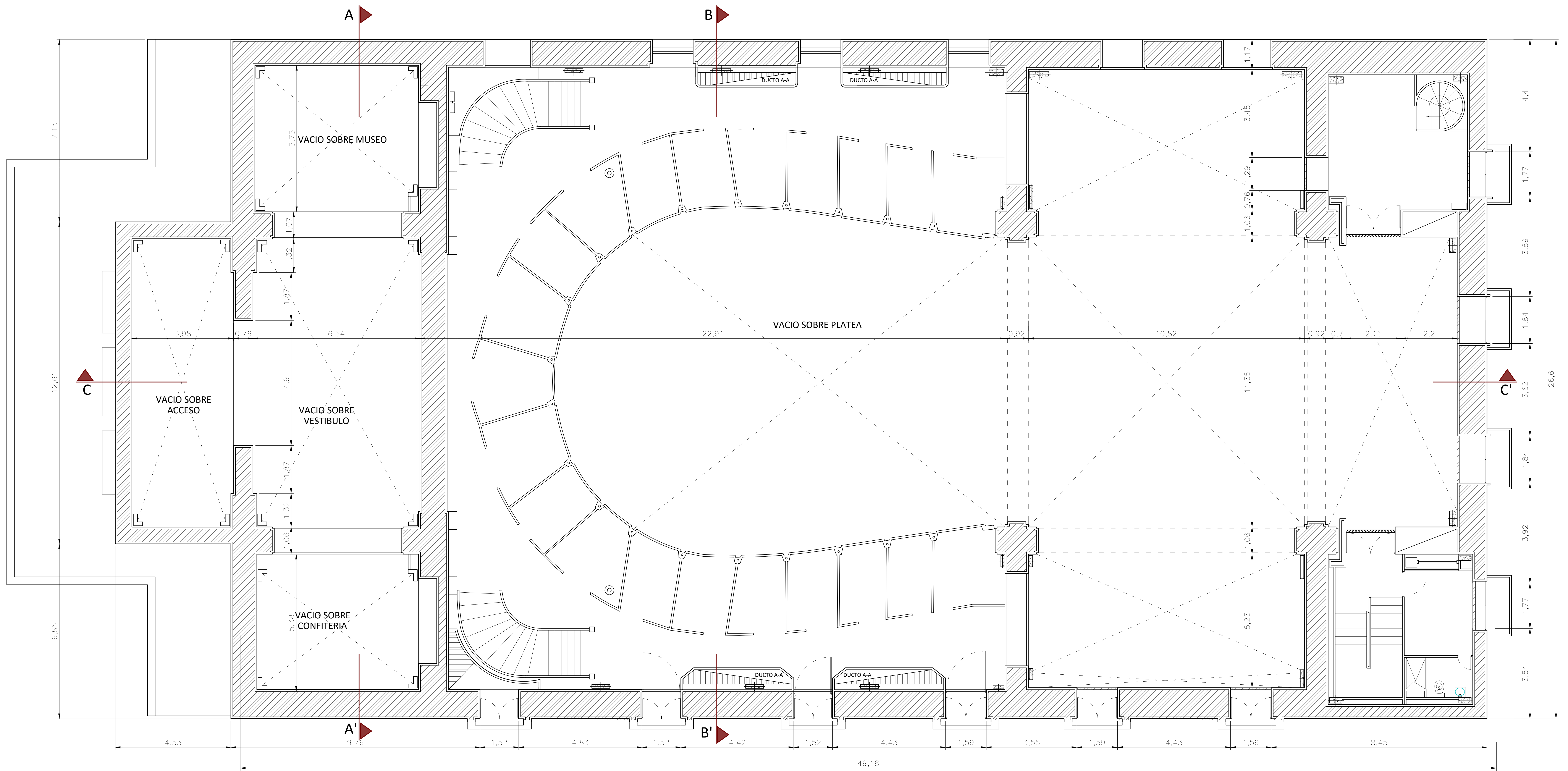
PLANTA ARQUITECTÓNICA SEGUNDO PISO Escala: 1:75
